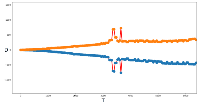
Fig. 6. : Phantom test
